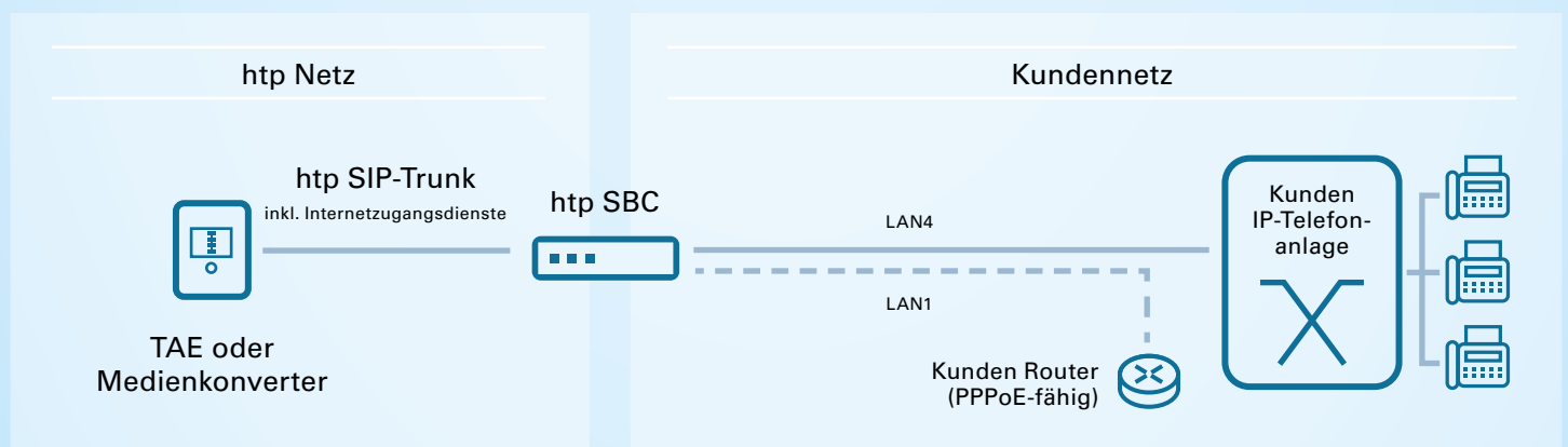
Abb.: SIP-Trunk Kundenanschlutung unter Verwendung eines kundeneigenen Routers
