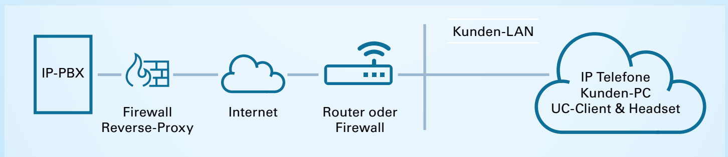
Abb.: Netzkonzept IP-PBX Internet-only
