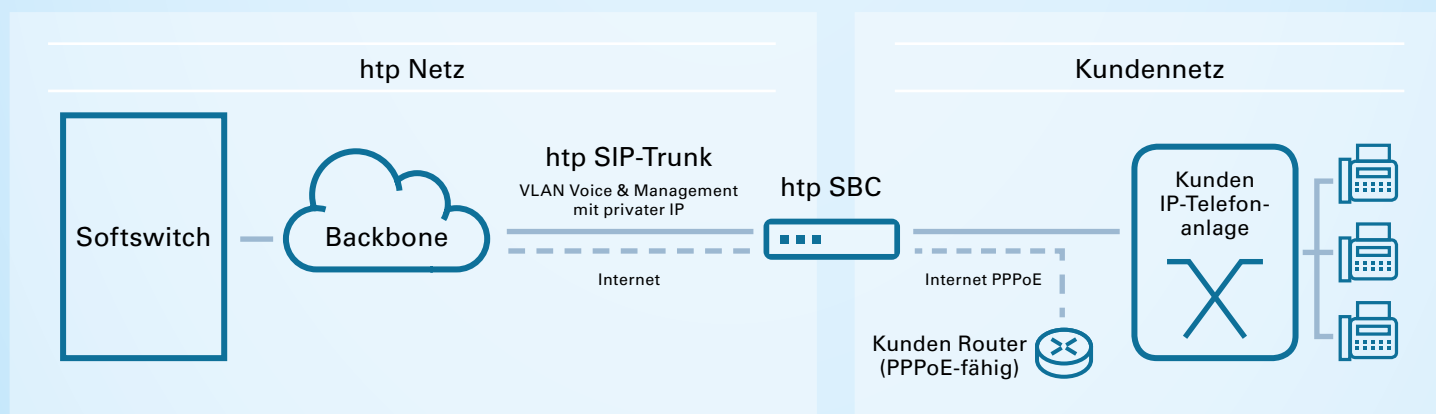
Abb.: SIP-Trunk Kundenanschaltung unter Verwendung eines kundeneigenen Routers
